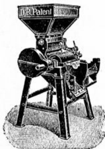
Schrotmühle
