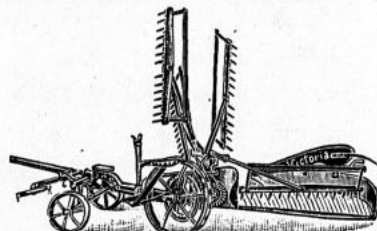
Viktoria-Getreidemaher mit Vordergestell.
