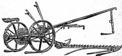
„Buckeye“ Grasmäher
