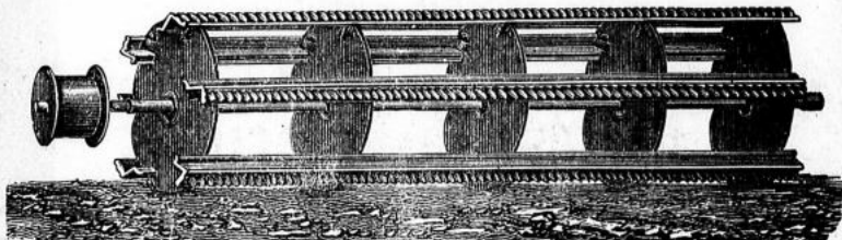
Neue Victoria-Dreschtrommel mit patentirten Stahlschlägeln
